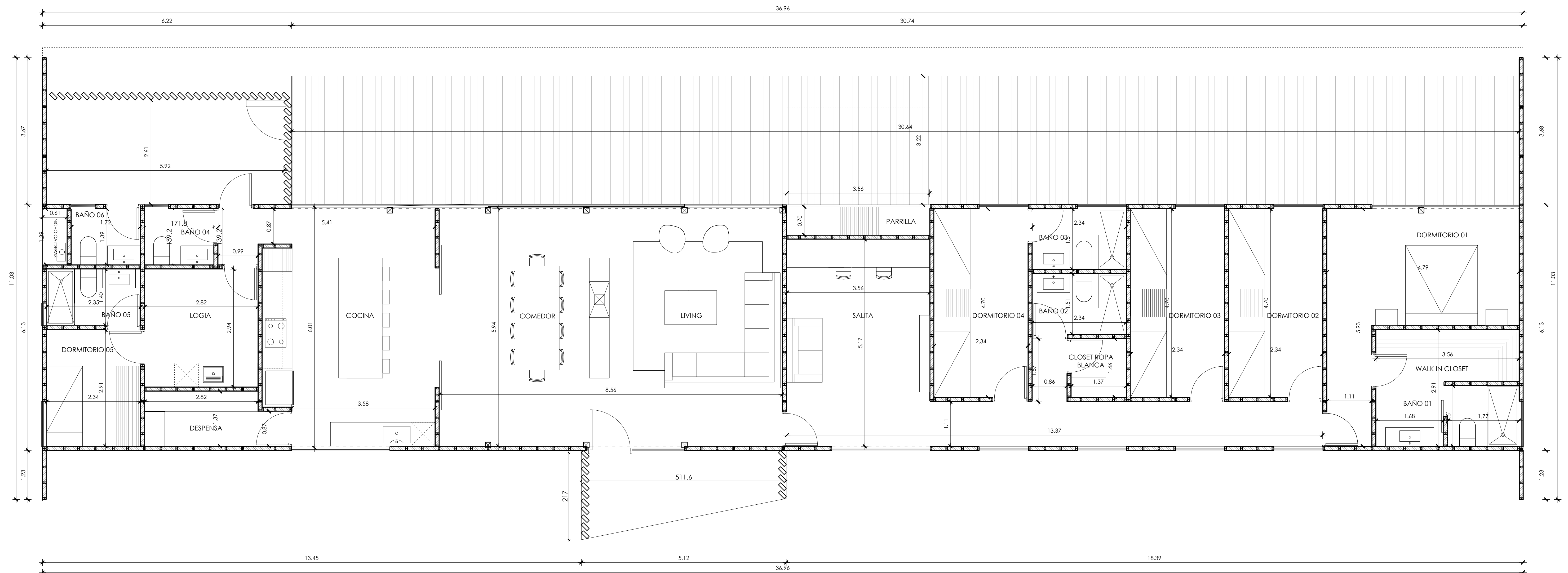
PLANTA ARQUITECTURA MEER 227
